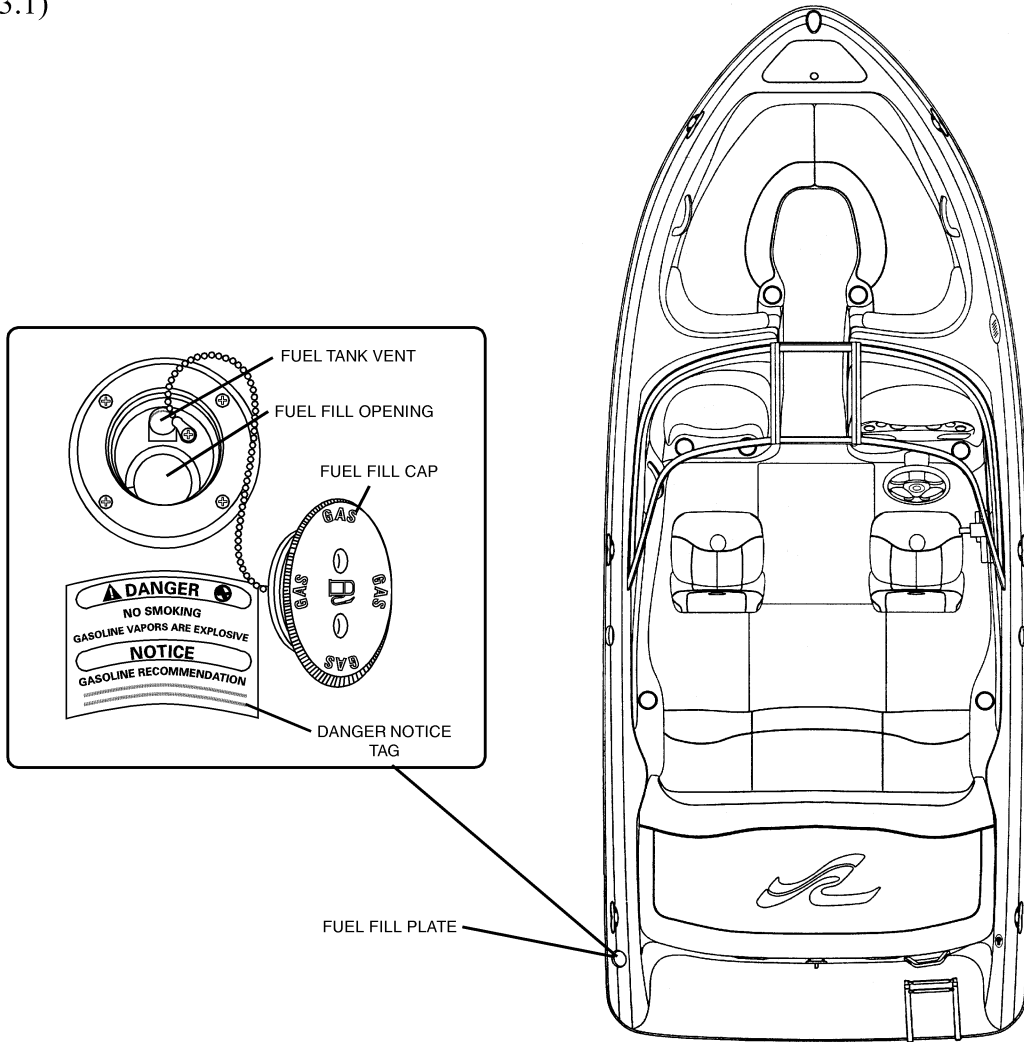
FUEL FILL LOCATION (FIG. 5.3.1)
