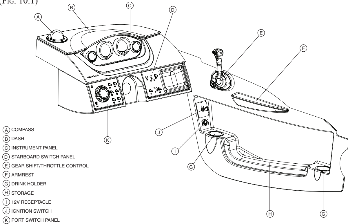
HELM LAYOUT (FIG. 10.1)
